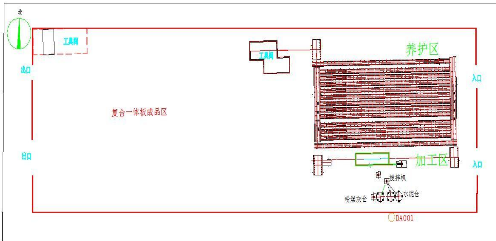
附图2-1 复合一体板生产车间平面布置图
