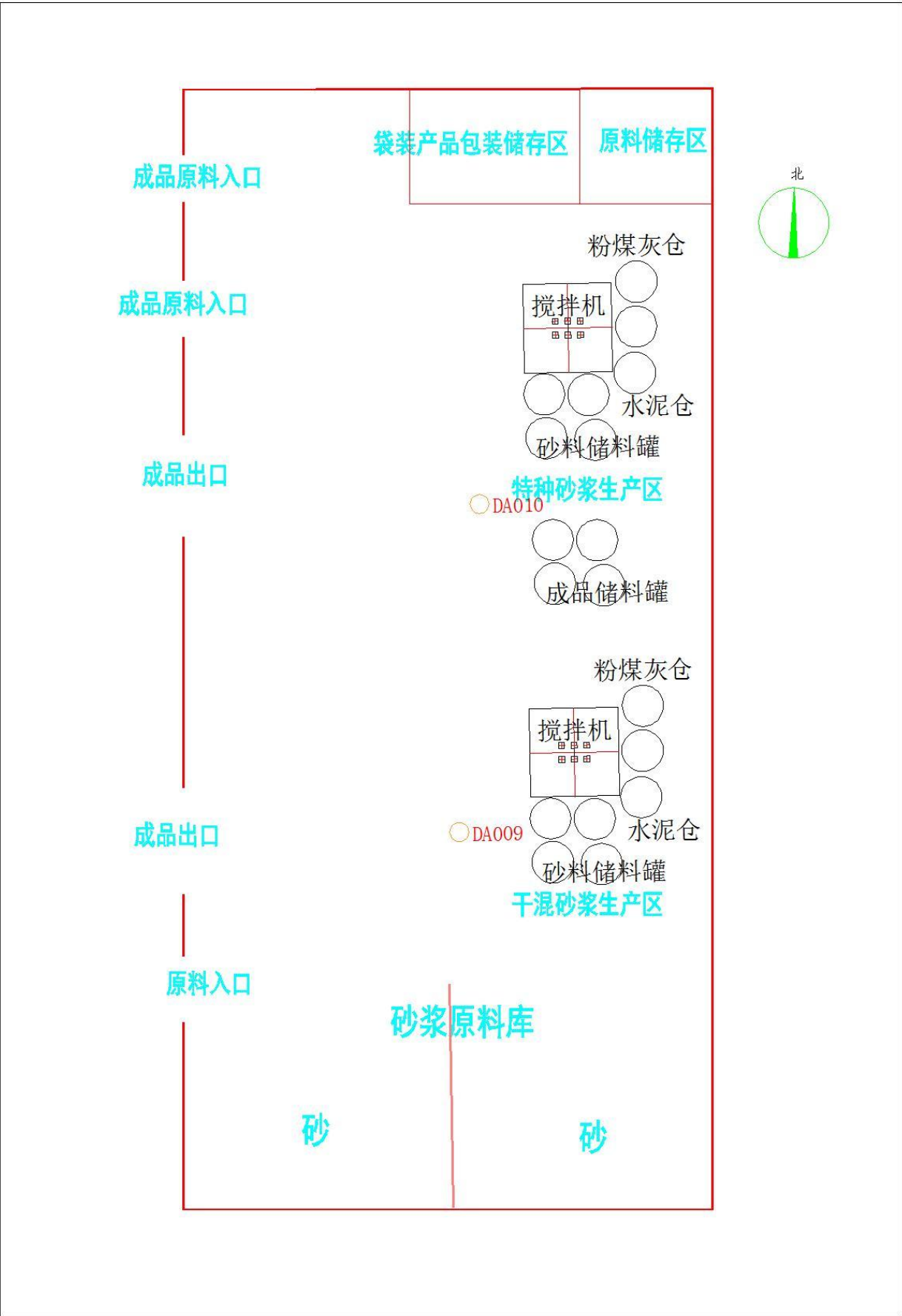
附图2-4 砂浆生产线平面布置图
