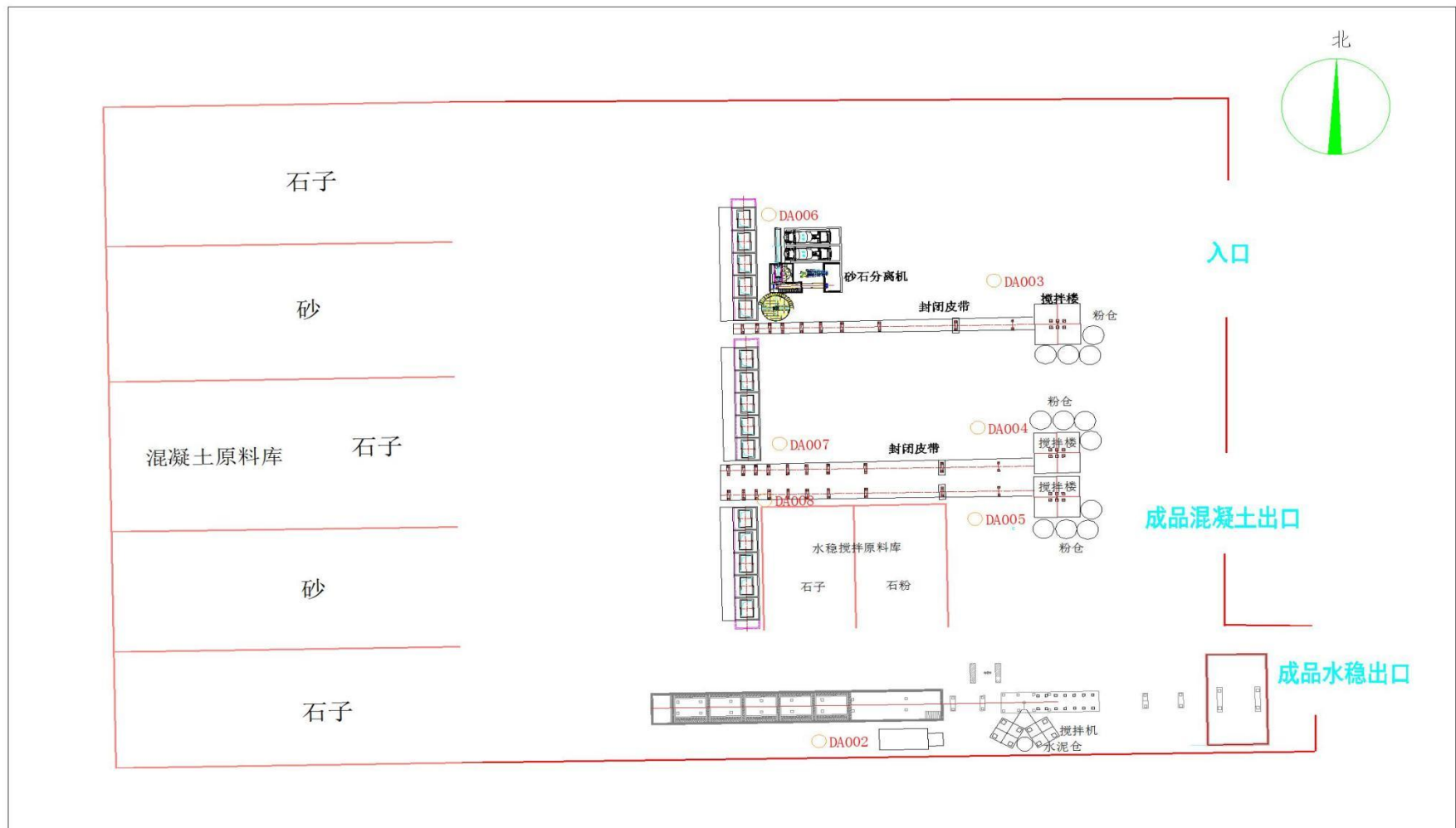
附图2-2 综合生产车间平面布置图
