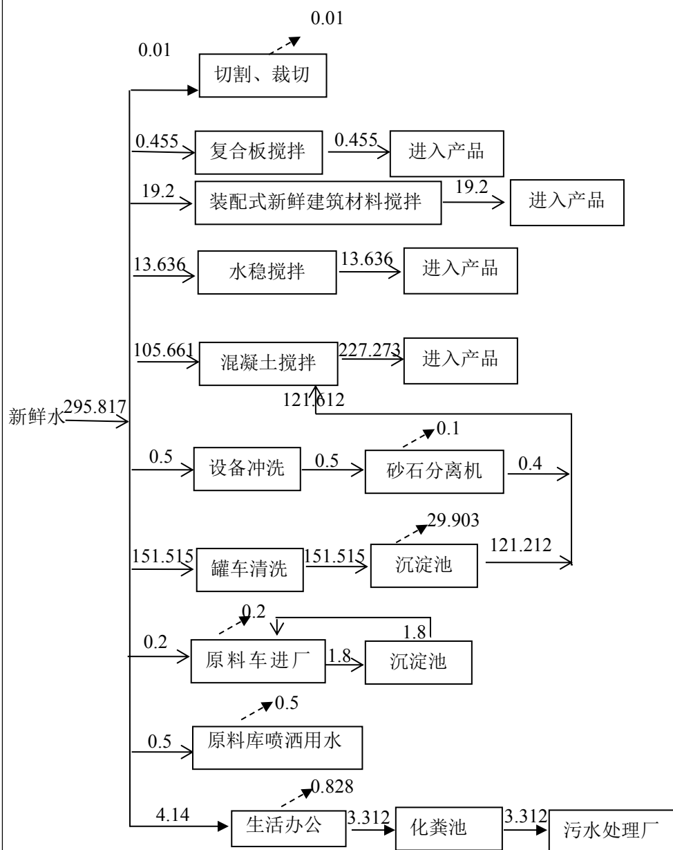
图 1 项目水量平衡图
